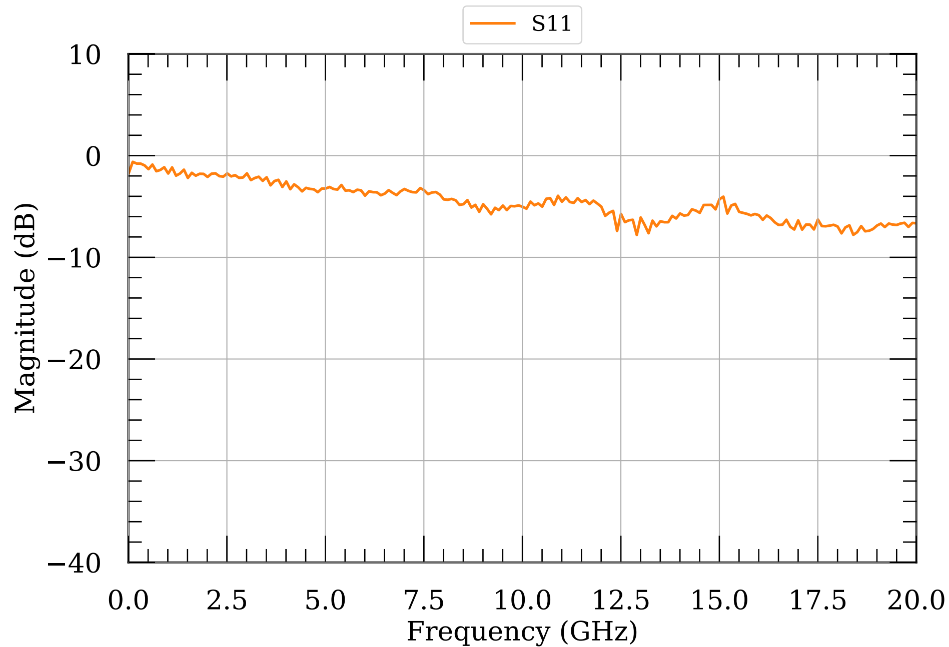
LNA S-params module033
